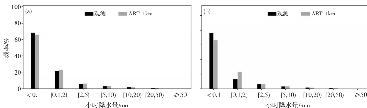
图4 2019—2022年5—8月广东20例暴雨过程中区域站(a)和水文站(b)的观测降水与 ART_1 km 降水在不同小时降水等级中的出现频率
