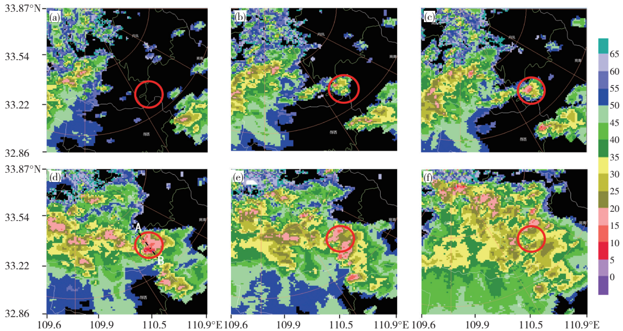
图2 2022年6月26日 11:17 (a)、11:39 (b)、11:45 (c)、12:30 (d)、12:47 (e)、13:13 (f)商洛多普勒天气雷达组合 反射率因子(单位: dBZ) (图2d中虚线AB为图3f商洛多普勒达径向速度剖面位置)
