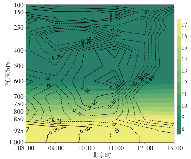
图8 2022年6月26日08:00—13:00金丝峡各层比湿(填色,单位: \text{g} \cdot \text{kg}^{-1} )及垂直速度(等值线,单位: \text{Pa} \cdot \text{s}^{-1} )演变
