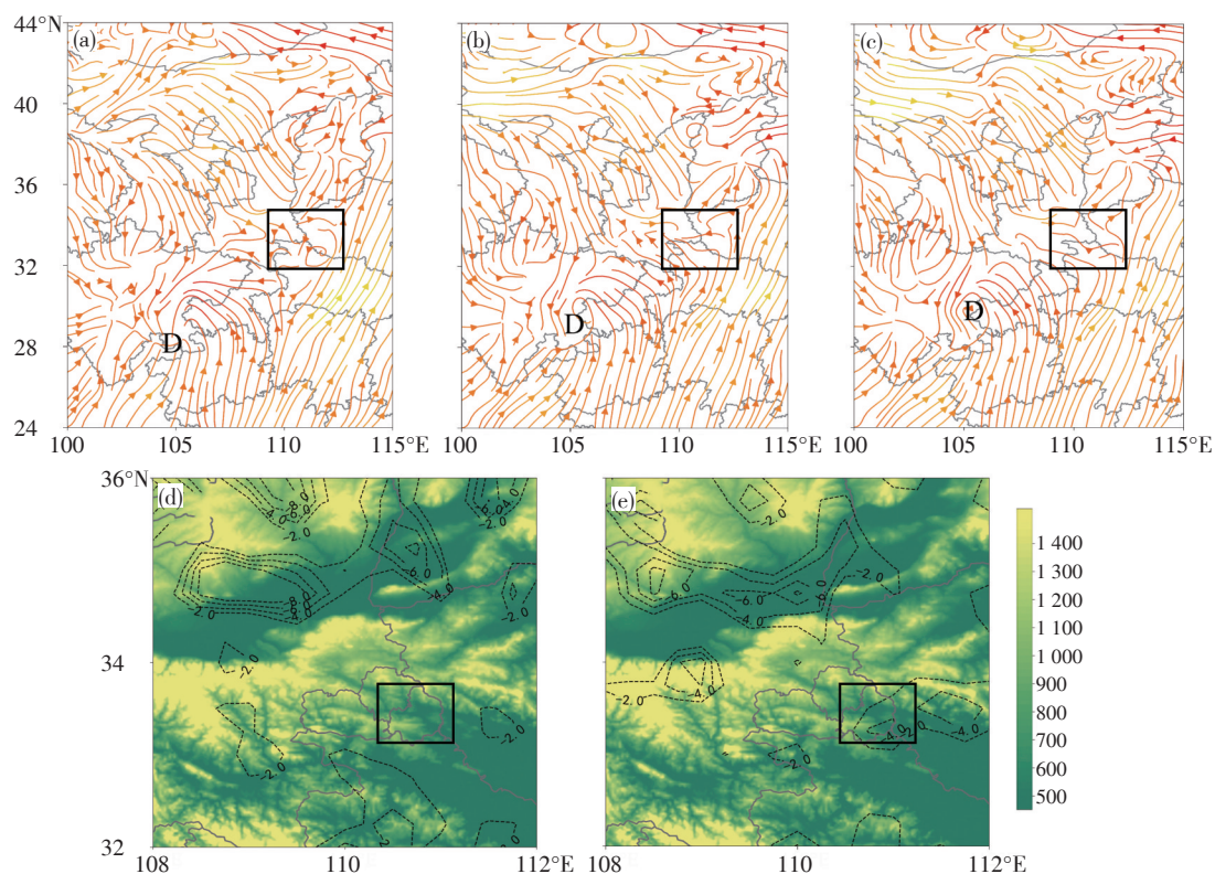
图 12 2022 年 6 月 26 日 09:00 (a)、10:00 (b)、11:00 (c)商洛 925 hPa 流场(单位: \text{m}\cdot\text{s}^{-1} )分布及 09:00 (d)、10:00 (e) 925 hPa 散度场(填色, 单位: 1 \times 10^{-5} \text{ s}^{-1} )和地形(填色, 单位: m)分布(D 代表低涡; 黑色方框为商南地区)
