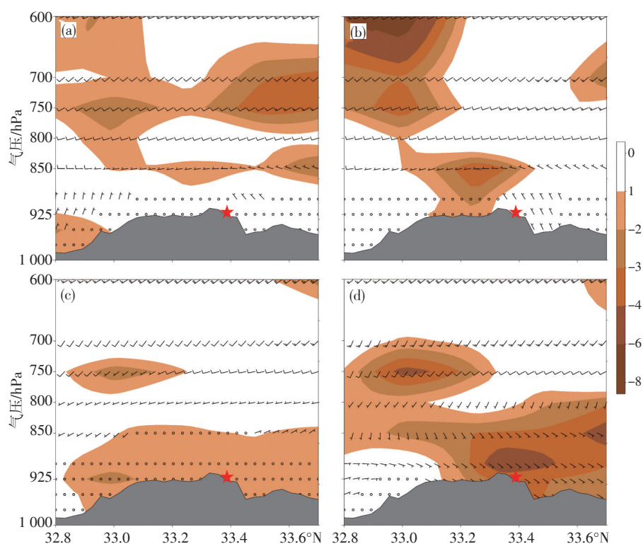
图 11 2022 年 6 月 26 日 08:00(a)、09:00(b)、11:00(c)、12:00(d)商南县风场(单位: \text{m}\cdot\text{s}^{-1} )、散度(填色, 单位: 1 \times 10^{-5} \text{ s}^{-1} )沿坐标( 110.32^\circ\text{E} , 33.25^\circ\text{N} )至( 110.83^\circ\text{E} , 32.83^\circ\text{N} )垂直剖面图
