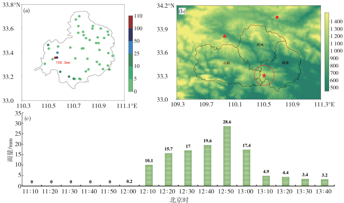
图1 2022年6月26日12:00—13:00商南县监测站累计雨量(a,单位:mm)、商洛地形分布(b,单位:m)、金丝峡站10 min雨量演变(c)(图b中红色圆圈为金丝峡地区,红色五角星为雷暴发生地,下同;红色实心圆为卢氏站探空位置,红色三角为商洛雷达位置)
