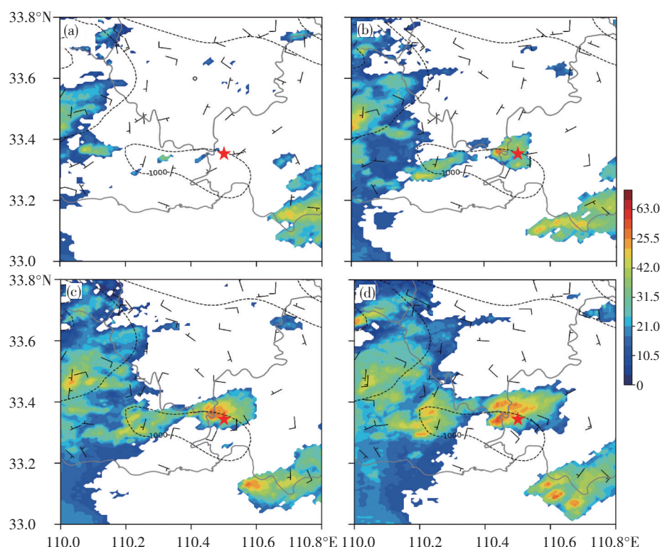
图10 2022年6月26日11:20 (a)、11:40 (b)、11:50 (c)、12:00 (d)商南地面风场(单位: \text{m}\cdot\text{s}^{-1} )及商洛雷达组合反射率因子演变(填色,单位: dBZ) (图中虚线为海拔高度1 000 m等值线)
