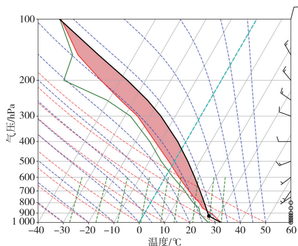
图6 2022年6月26日12:00金丝峡大气垂直结构
