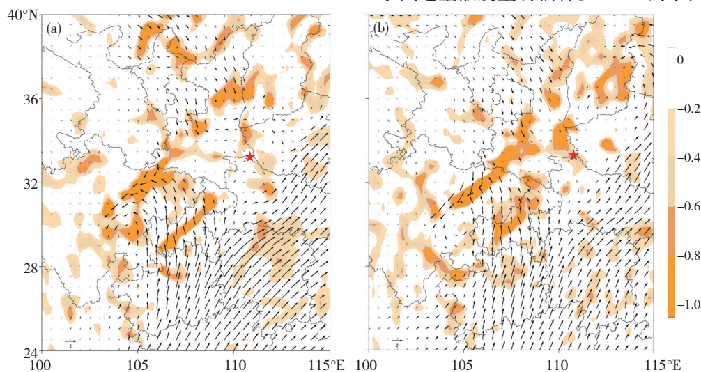
图7 2022年6月26日08:00(a)、12:00(b)商洛850 hPa水汽通量(箭头,单位: \text{kg} \cdot \text{s}^{-1} \cdot \text{hPa}^{-1} \cdot \text{m}^{-1} )及水汽通量散度(填色,单位: 10^{-7} \text{ kg} \cdot \text{s}^{-1} \cdot \text{hPa}^{-1} \cdot \text{m}^{-2} )分布
