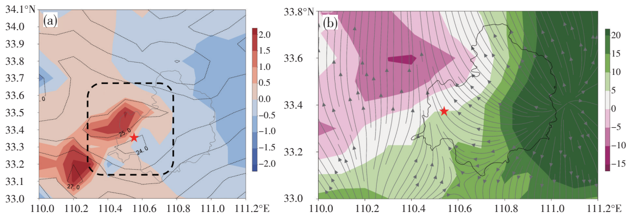
图9 2022年6月26日11:00地面2 m温度场(填色,单位: ^\circ\text{C} )及1 h变温(等值线,单位: ^\circ\text{C} ) (a), 3 h变压场
