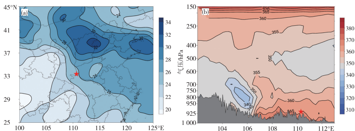
图5 2022年6月26日12:00 850 Pa与500 hPa温度差值场(a,单位: °C)及12:00沿33.25°N
